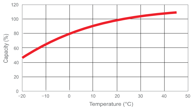
CAPACIDAD VS TEMPERATURA
