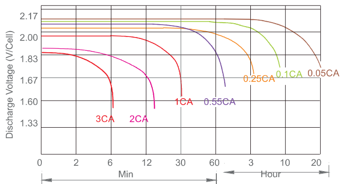
CARACTERÍSTICAS DE DESCARGA (25°C)
