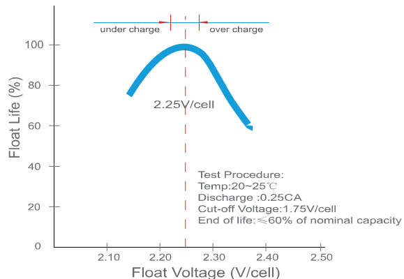
ESTACIONARIO/ CARACTERÍSTICAS FLOTACIÓN
